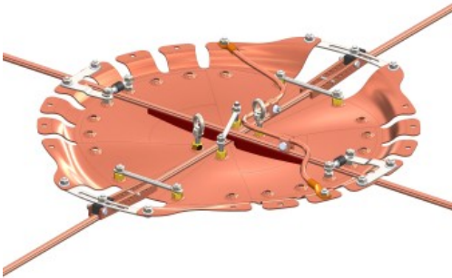
Die neue Fahrdrabtkreuzung (konstruktive Anpassungen vorbehalten)
