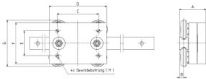
Schnittdarstellung der IBC FLEXY-Runner Kurvenführung
